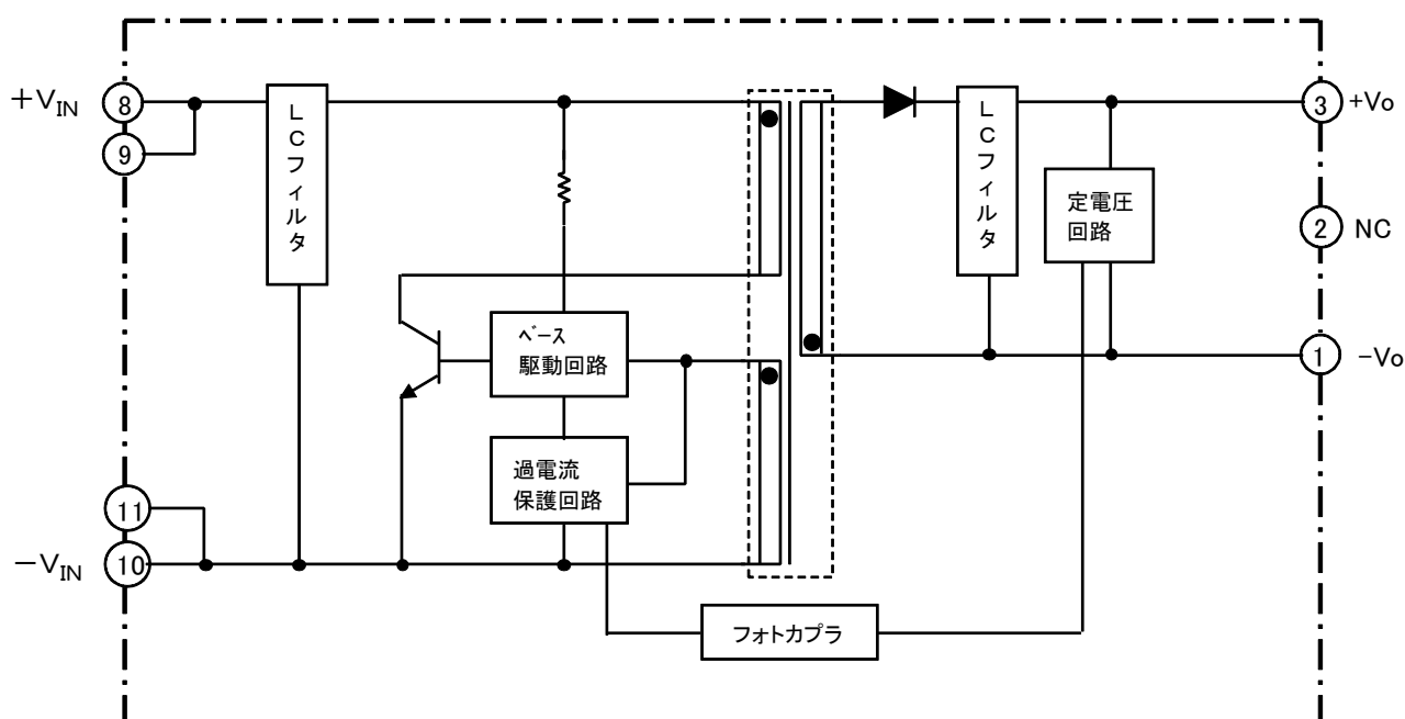
ブロック図
