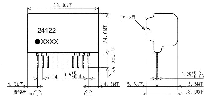
外形図
