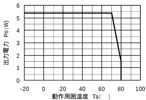
ディレーティング曲線 ( V_i=220 \sim 410V )
