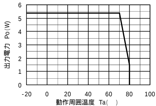
ディレーティング曲線 ( V_i=220 \sim 410V )
