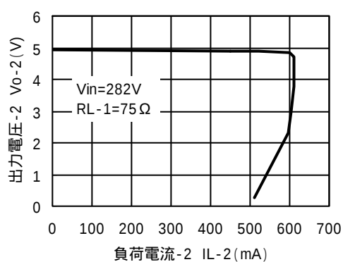
出力電圧-負荷電流特性-2 (代表例)
