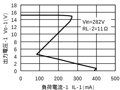
出力電圧-負荷電流特性-1 (代表例)
