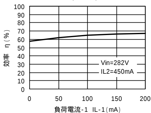
効率-負荷電流特性-1 (代表例)
