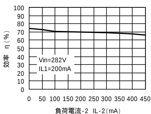
効率-負荷電流特性-2 (代表例)
