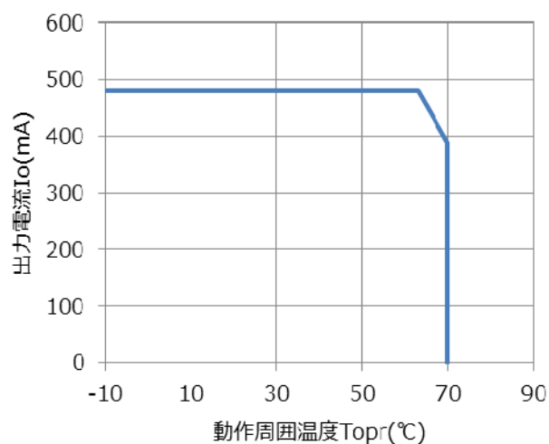
デレーティング特性
