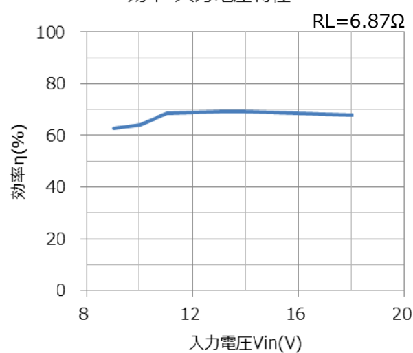
効率-入力電圧特性
