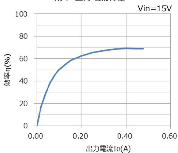
効率-出力電流特性
