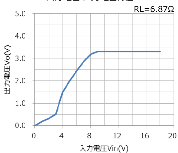
出力電圧-入力電圧特性
