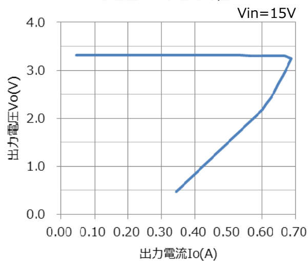
出力電圧-出力電流特性
